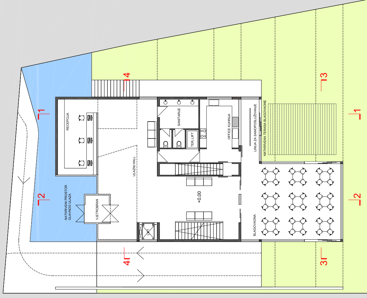
TLOCRT PRIZEMLJA 1:100
