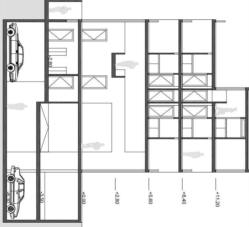
PRESJEK 4-4 1:100
