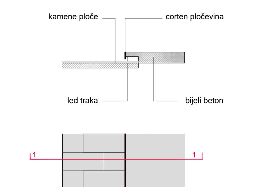
DETALJ SPOJA POZORNICE S OPLOČENJEM PODA
