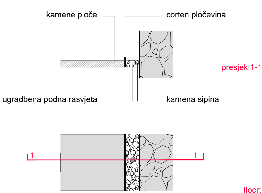
DETALJ SPOJA KAMENIH ZIDINA S OPLOČENJEM PODA
